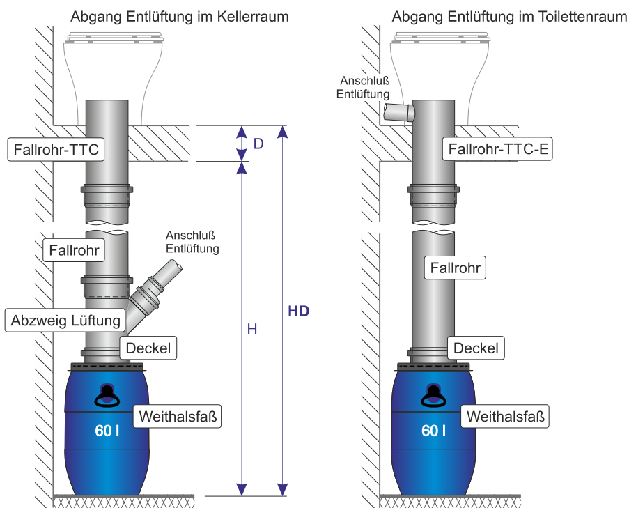
Auswahltabelle für Fallrohre, nach Deckenstärke, Raumhöhe und Lüftungsabgang
